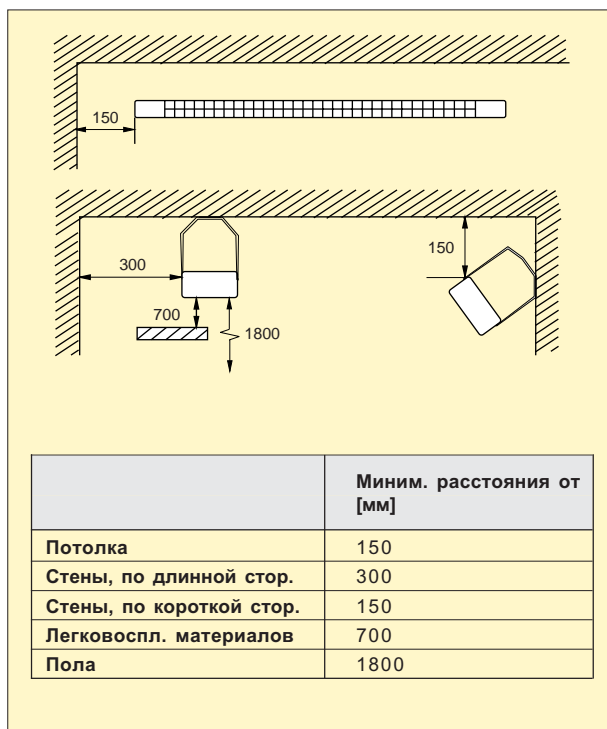
Рисунок 3: Минимальные расстояния при стационарной установке.
